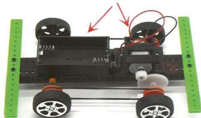
粘贴电池盒，导线连接电机
