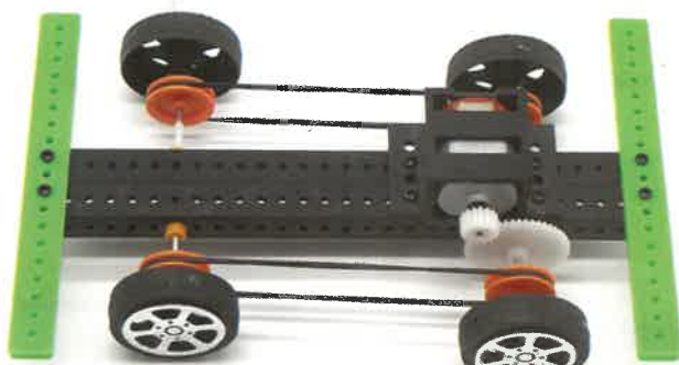
螺丝、螺母分别将绿条中间位置固定在黑条第1个孔上
