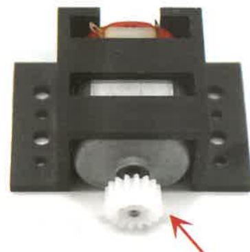
电机放到电机座里，齿轮按压在电机轴上
