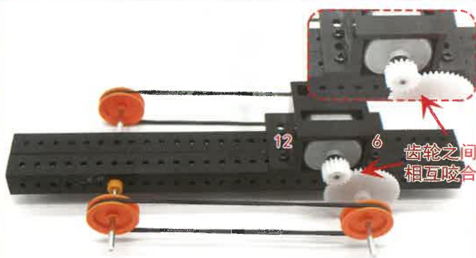
螺丝、螺母将电机座固定在黑条第6、12个孔上
