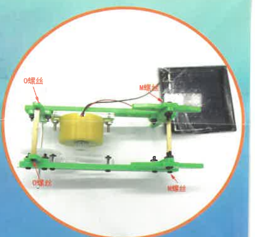
6. 将齿轮轴I安装到A板绿色十字条的孔里, 用黑色螺丝M将铜柱固定在A板上, 如图所示
