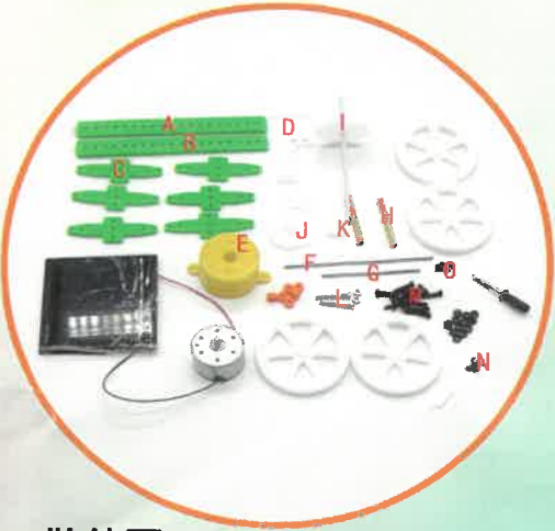
1. 散件图
