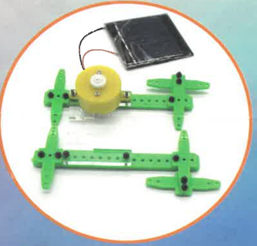
4. 用黑色螺丝M将D板安装到A板和B板上, 再用银色螺丝L将电机座固定在D板上, 如图所示
