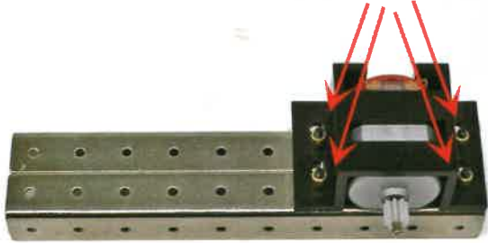
用螺丝与铜柱将电机座固定在车架上 3
