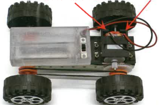
粘贴电池盒，并连接电机 8
