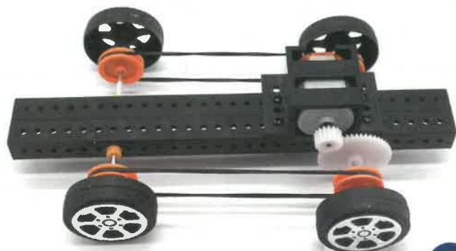
安装车轮
