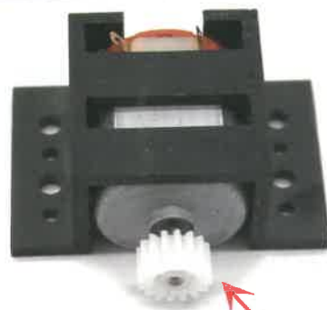
电机放到电机座里，齿轮按压在电机轴上
