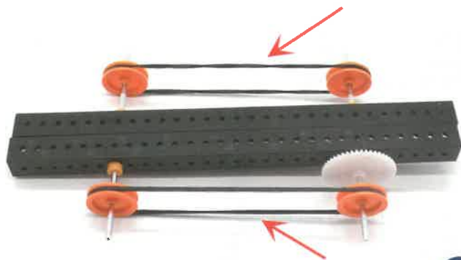
安装皮带
